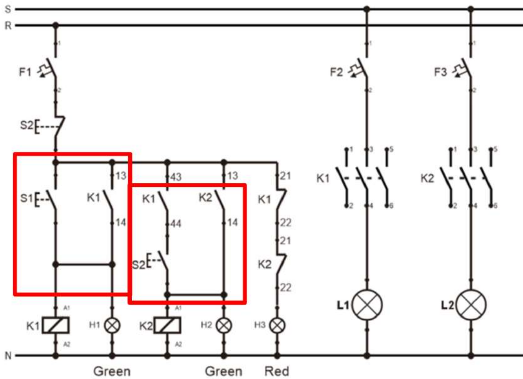
JOB ORDER 6 KENDALI MOTOR MENYALA BERURUTAN (MANUAL)
